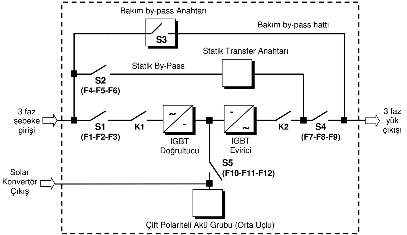
Şekil 1.1 DS300HYB Serisi UPS Blok Şeması
